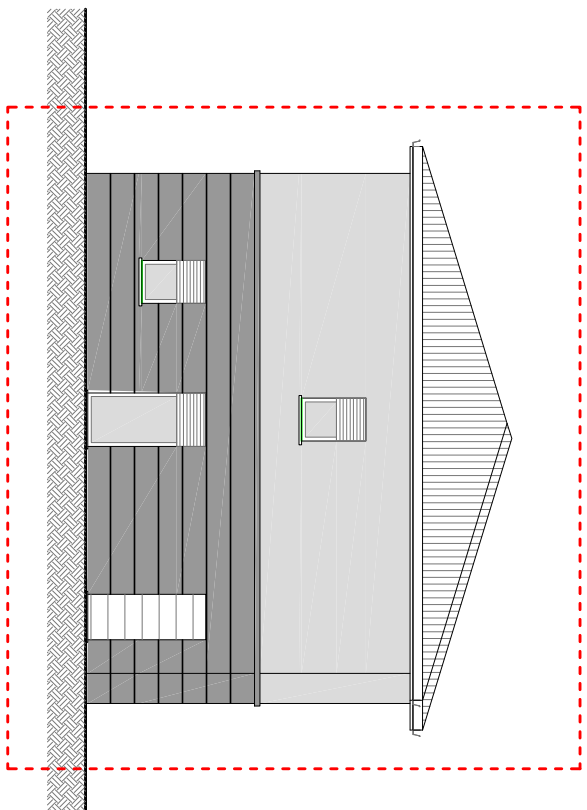
PROSPETTO FIANCO EST
