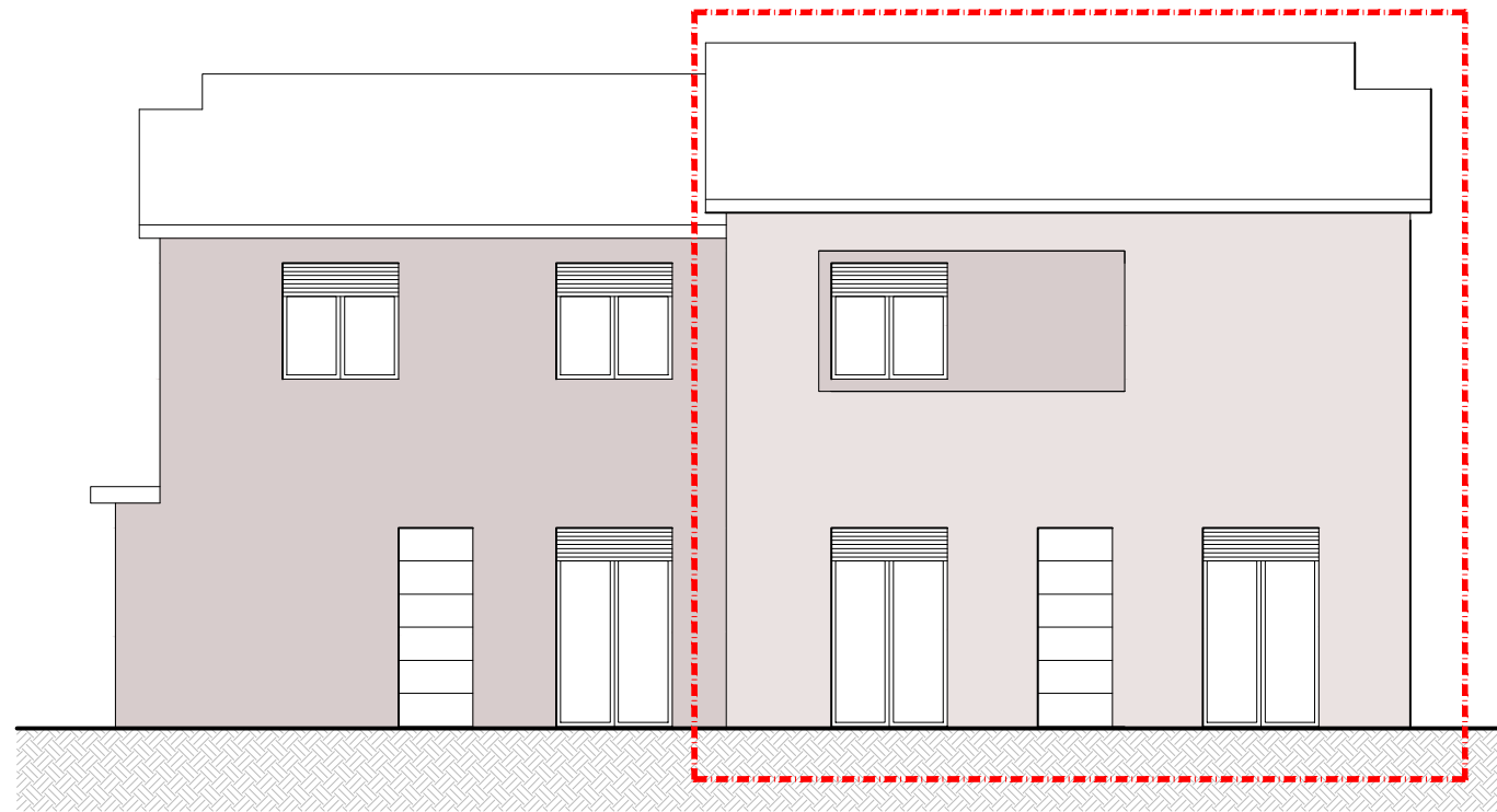
prospetto fronte villetta n. 1
