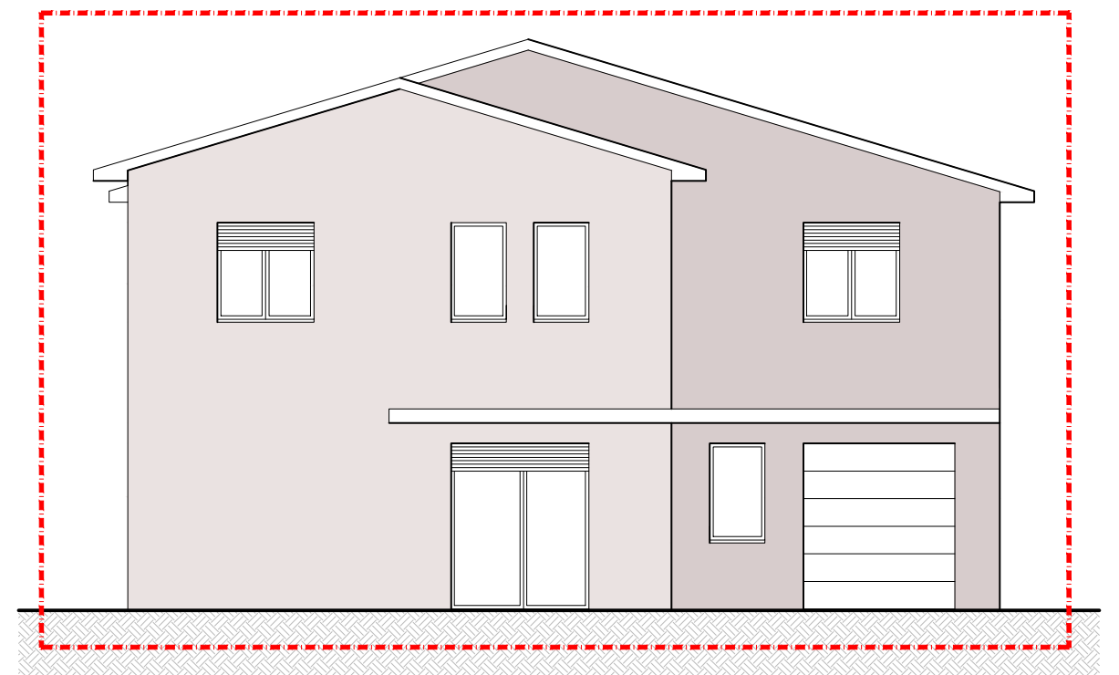
prospetto fianco villetta n. 1
