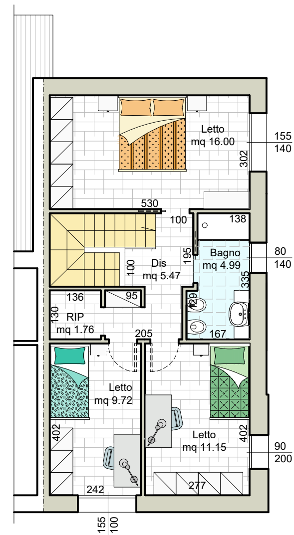
Piano primo
