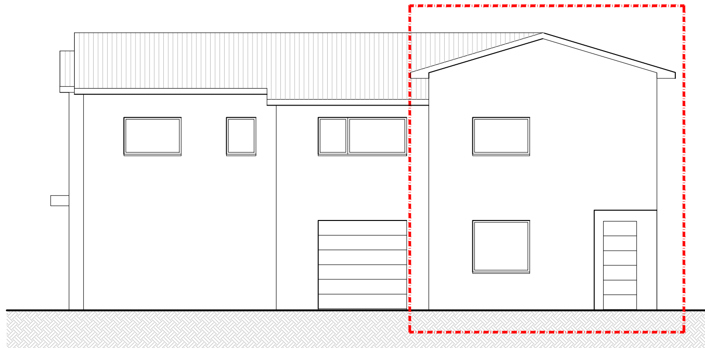
Prospetto fronte
